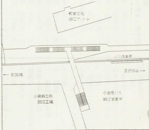
横断歩道橋新設工事平面図
